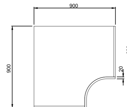
Base concava curva 900x900 e pensile concavo curvo 600x600 Internal curved base and wall units Вогнутые нижняя тумба и навесной шкаф
