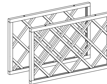
COPPIA GRIGLIA PORTABOTTIGLIE WINE RACK INSERT (PAIR) пара решеток для бутылок 335 x 567 x 20
