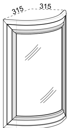
VETRINA CURVA "H" = 956 - 716 CURVED GLASS DOOR Рамка закругленная
