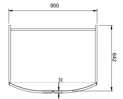
Coppia ante curve Curved doors (pair) Пара гнутых дверок
