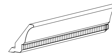
CORNICE COPERCHIO CON DECORO CORNICE MOULDING WITH DECORATION Карниз с декором 3000 x 119,6 x 30
