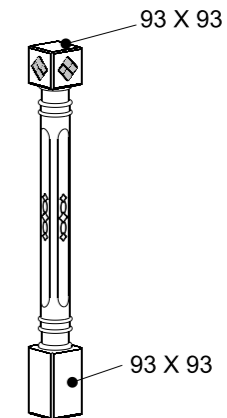
GAMBA ISOLA C/DECORO LEG FOR PENINSULA ножка островная с декором "H" = 870
