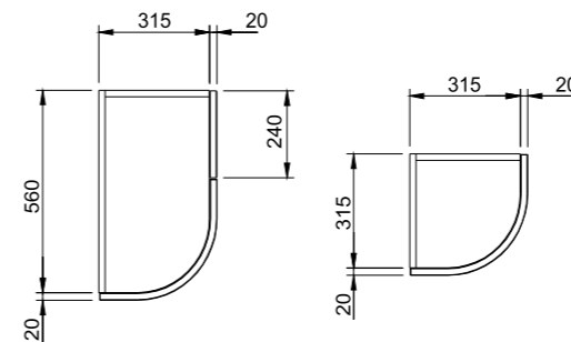
Terminali base e pensile Base and wall units Закругленные нижняя тумба и навесной шкаф
