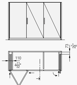
Передні фасади шаф з підлоговим профілем
