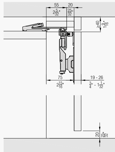
Покриття ніши без меблевої поверхні
