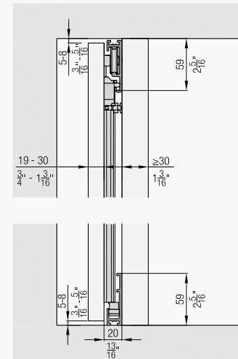
Двері від підлоги до стелі, гардеробна
