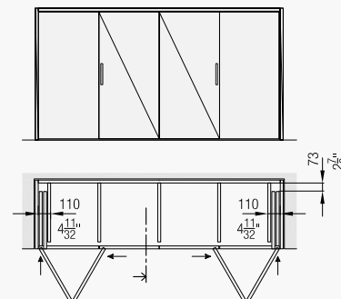
Покриття ніши без меблевої поверхні
