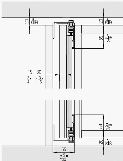
Двері опираються в полку і верхню частину шафи
