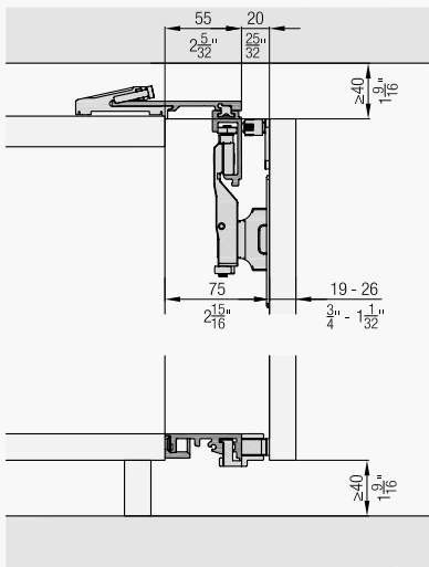
Передні фасади шаф з підлоговим профілем
