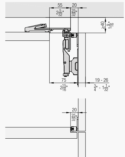
Версія половинної висоти зі стільницею
