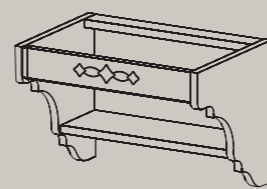
SOTTOPENSILE MIDWAY UNIT 315 x 900 x 315 - 315 x 450 x 315
