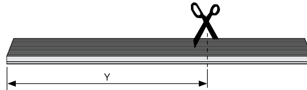
Barra di collegamento superiore - Section drawing connecting bar for upper sliding units - Oberer Verbindungsstange - Profilé de connexion supérieur - Sección de corte de la pieza de union carril superior
