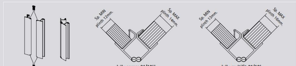
A. Giunzione Junction
