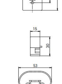
Gancio a molla Spring clip
