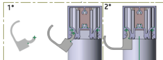
МОНТАЖ АКЕСУАРІВ
