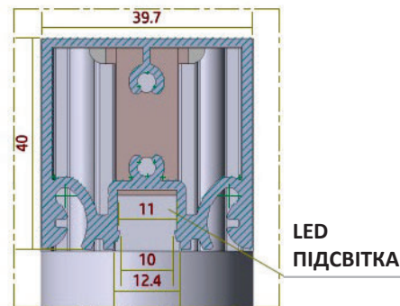
МОНТАЖ АКЕСУАРІВ
