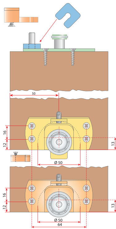
CUSCINETTO Ø 30
