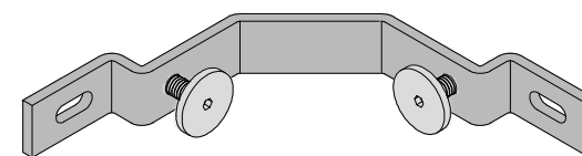
Attacco e regolazione angolo Wall Corner Fixing and Setting 3PC008
