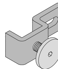
Attacco e regolazione a muro Wall Fixing and Setting 3PC002
