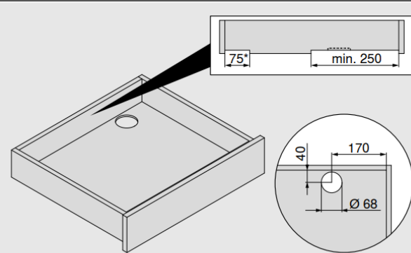
Розетка – Шухляда з ДСП MOVENTO
